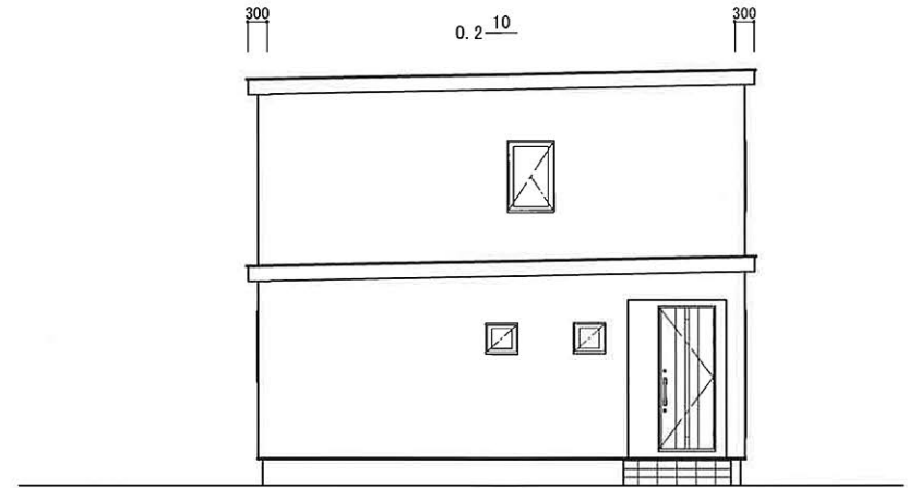
東側 立面図 S:1/100
