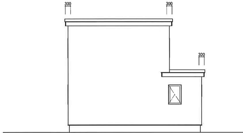
南側 立面図 S:1/100
